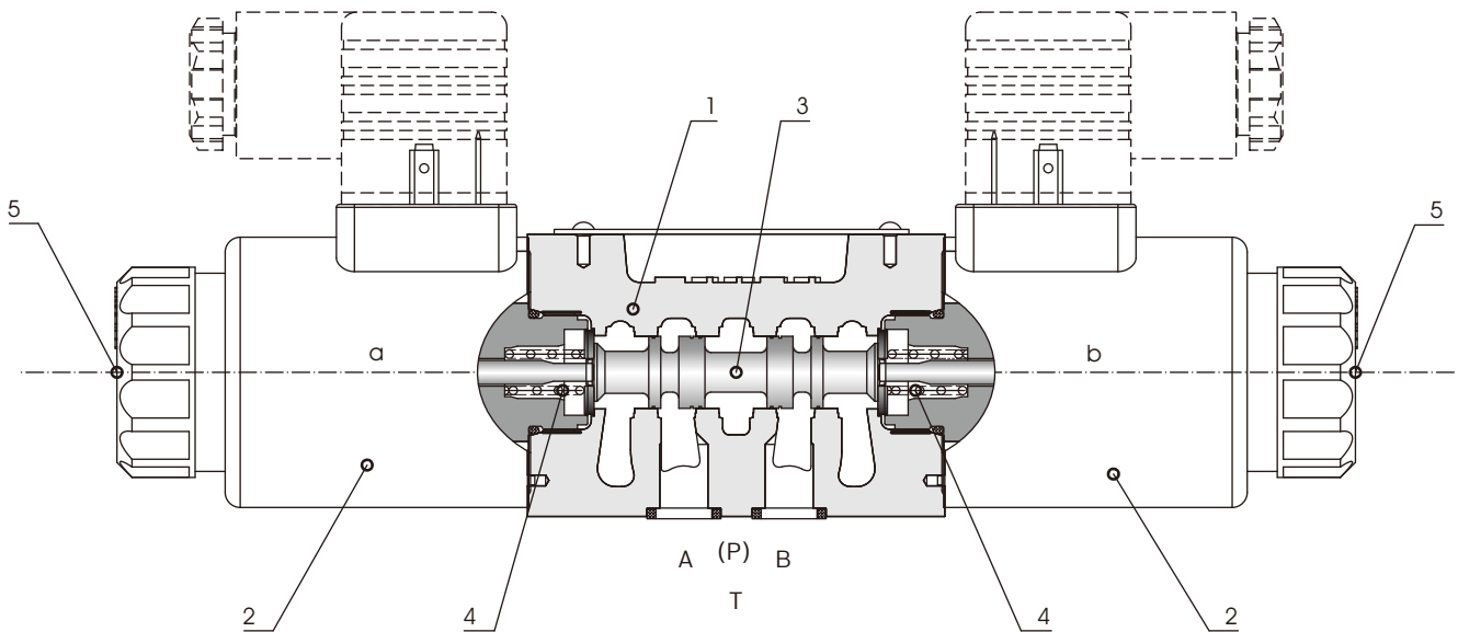
型号 4WE 6 E LX1/E...
