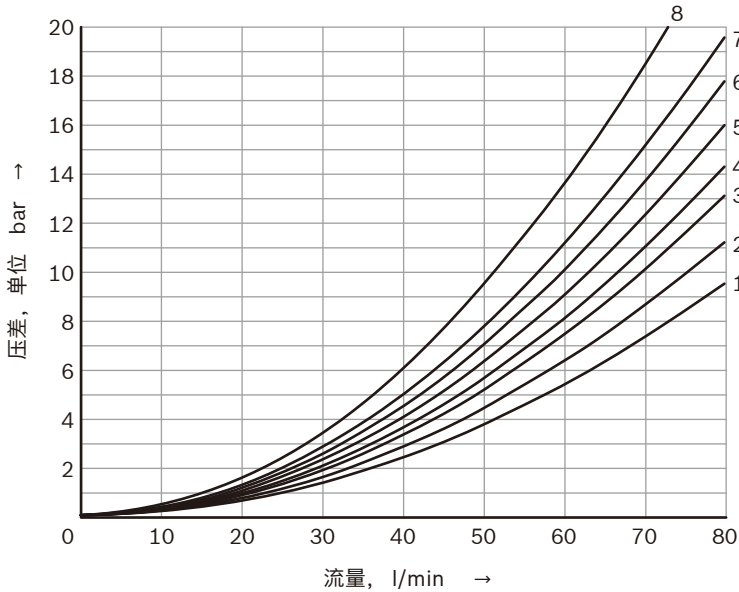
\Delta p - q_v 特性曲线
